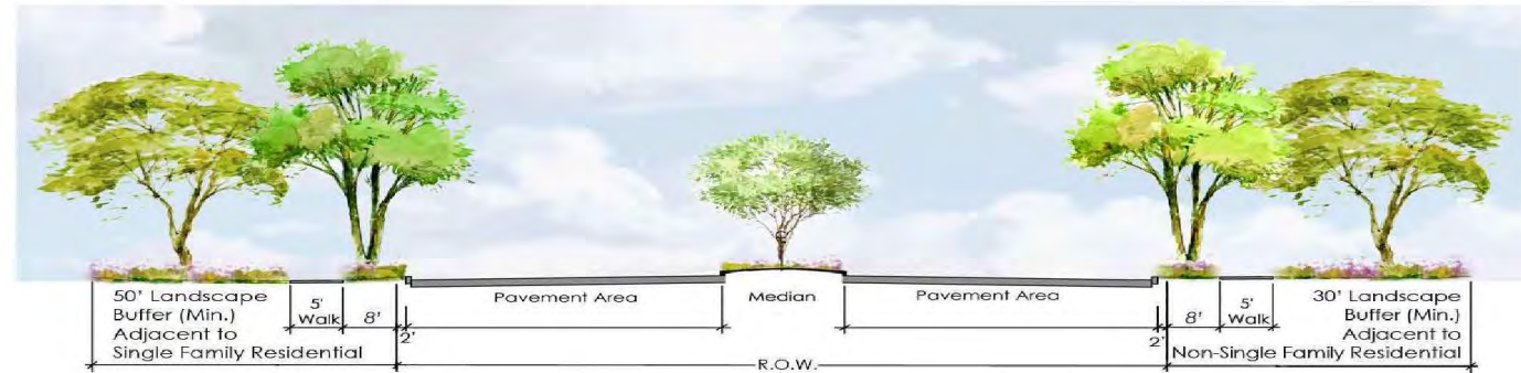
■■■■■■■■■■ Foothills Principal Arterial Section
