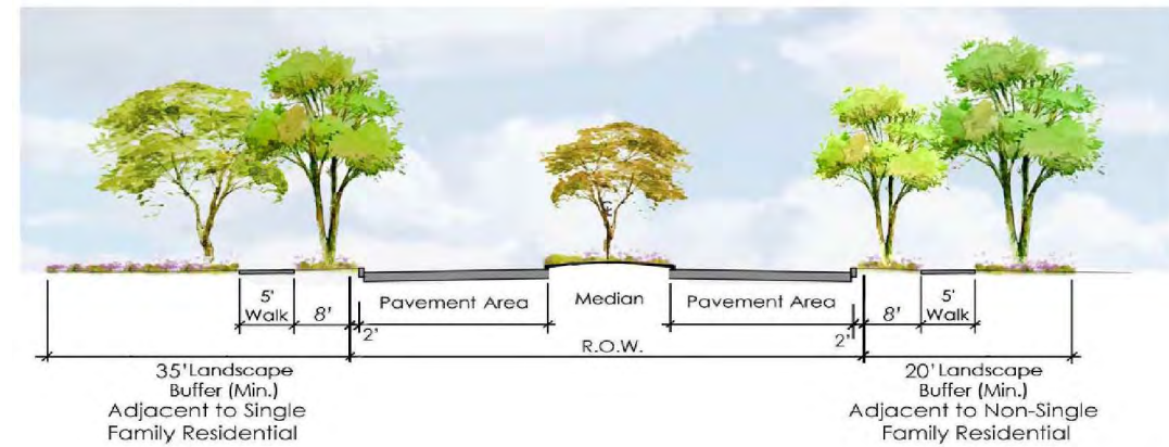
■■■■■■■■■■ Collector Street Section
