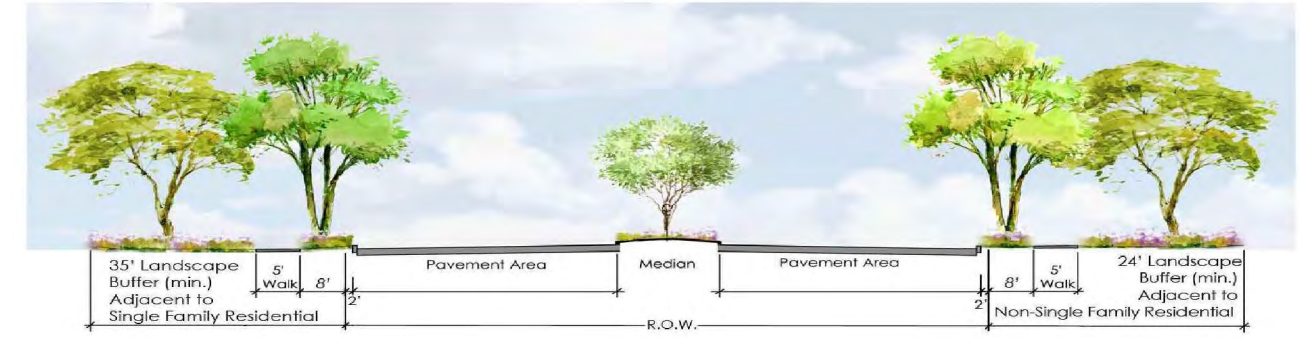
■■■■■■■■■■ Foothills Minor Arterial Section
